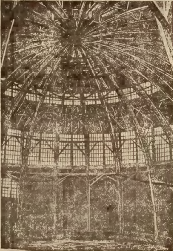
Wnętrze dancingu. — Projekt inż. arch. J. Müllera. Konstrukcja: pełne węzary łukowe z desek; rozpiętość wolna 30 m. wysokość 18 m. Największa kopuła drewniana w Europie.
