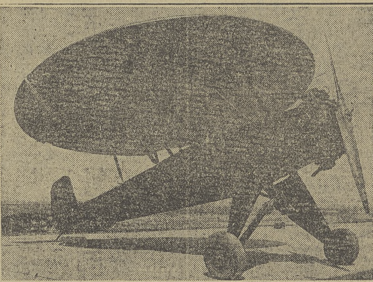
Model nowego samolotu, ze skrzydłem w formie wielkiego parasola, który może lądować na płaszczyźnie o średnicy 25 stóp, a więc na przeciętnym podwórku za domem. Samolot wywijał się szybkość 135 mil na godzinę i lądował powolniej, niż spadochron. Pomysłne próby przeprowadzono na lotnisku Curtissa.
